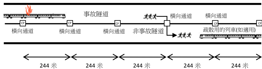
圖二：顯示地下及密封軌道內的橫向通道 之間的最大距離為 244 米的簡圖
