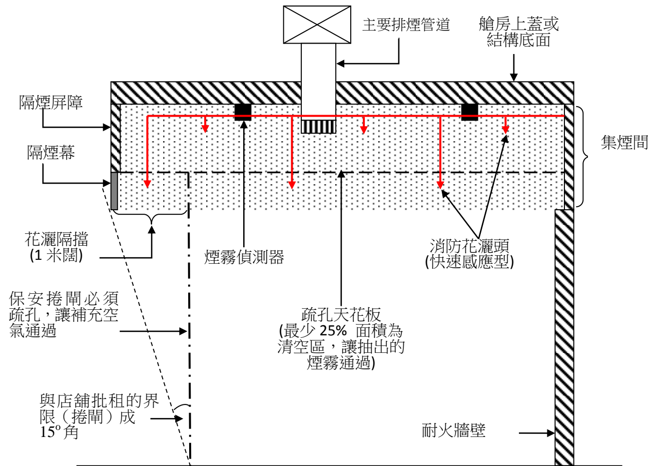
圖五：「艙房概念」的簡圖
