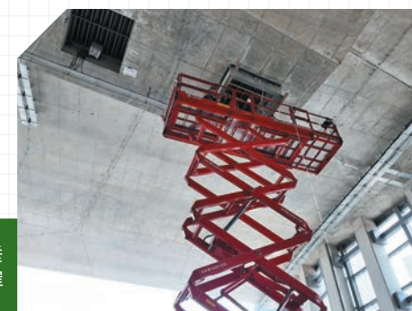
中九龍幹線工程團隊研發「垂直風罩測量設備」，快速並準確地測量排煙系統的風速。
